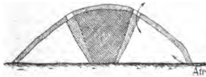
Fig. 16. — Marche de la carbonisation dans une meule circulaire.
